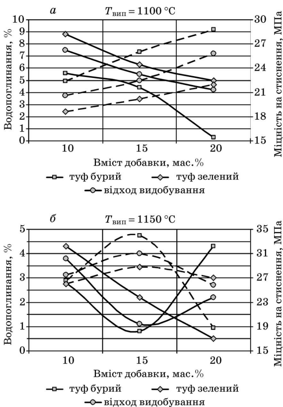
Рис. Залежності водопоглинання (—) та міцності на стиснення (- -) зразків, випалених за 1100 °С (а) та 1150 °С (б), від вмісту добавки
