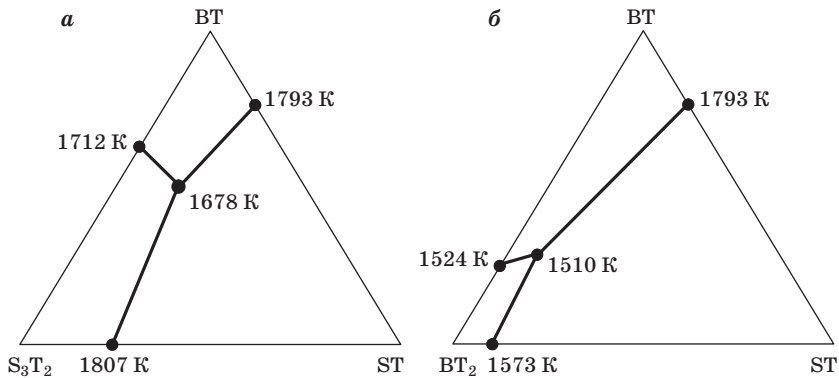
Рис. 2. Кривые ликвидуса тройных сечений:
